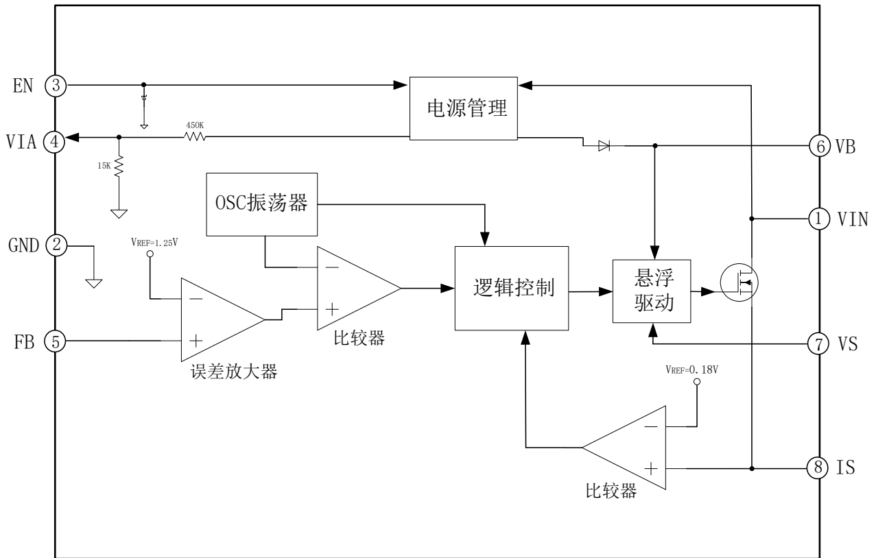
图 5-1. EG1192S 内部电路图
