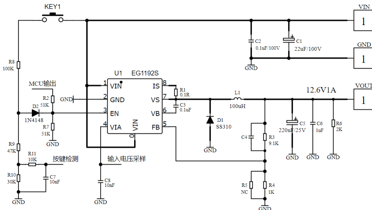
图 6-1. EG1192S 按键使能零功耗控制典型应用图
