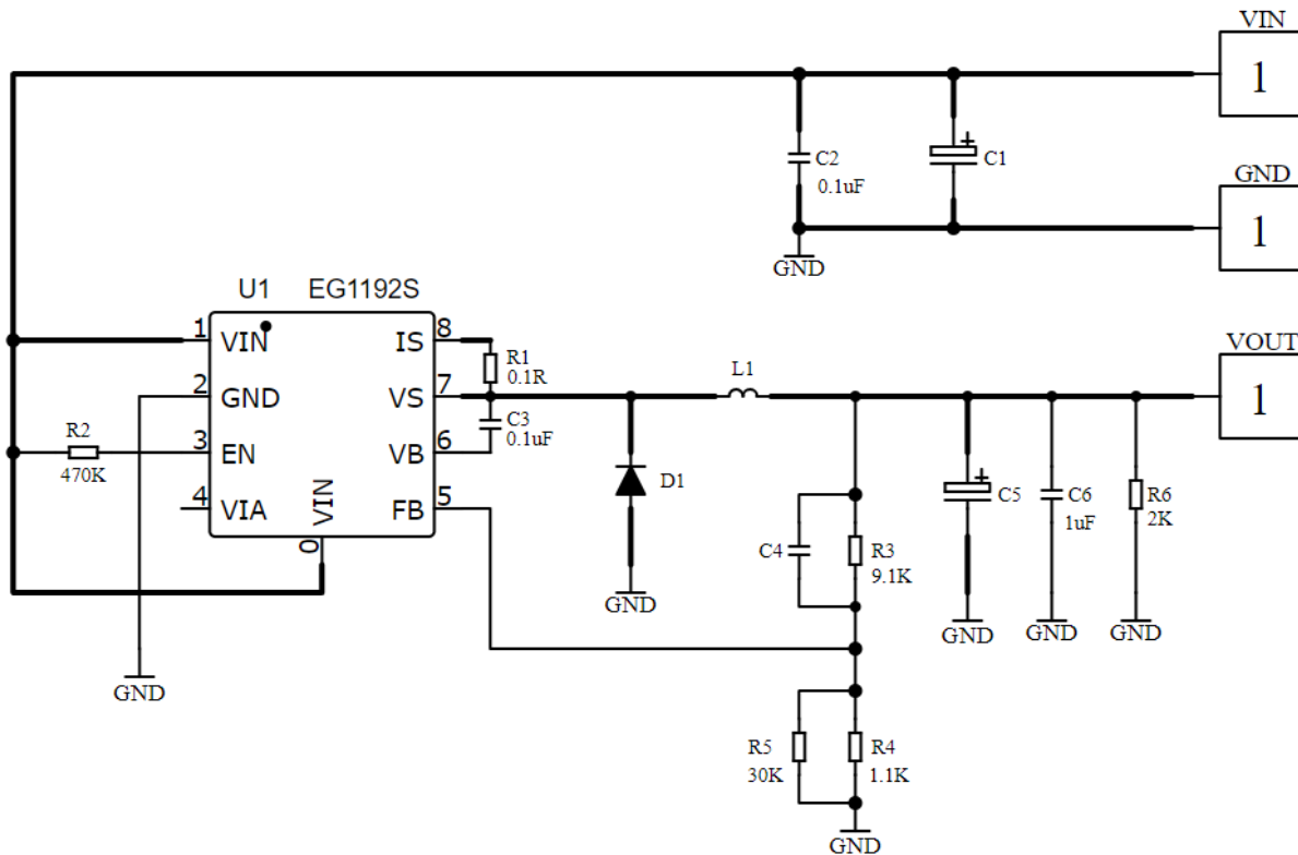
图 6-2. EG1192S 12V 输出典型应用图
