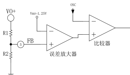
图 8.5 EG1192S 输出电压调整电路
