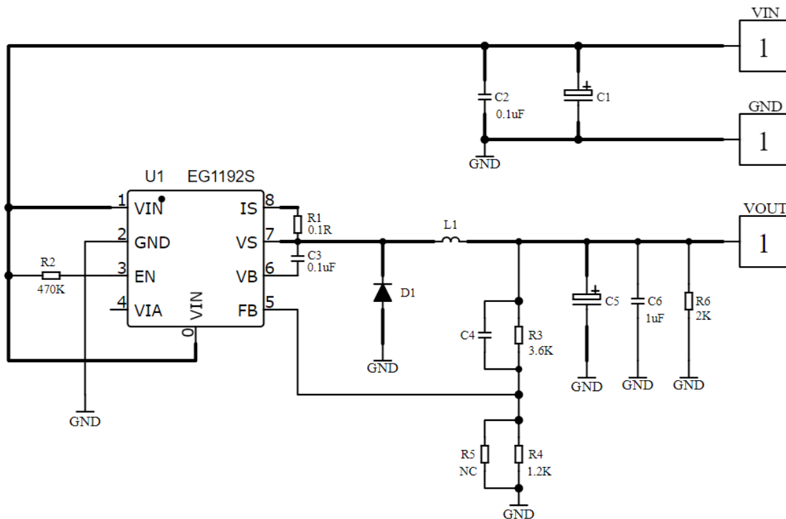
图 6-3. EG1192S 5V 输出典型应用图
