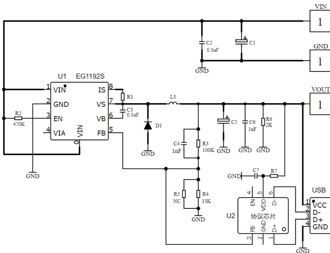
图 6-4. EG1192S 快充方案典型应用图
