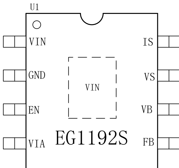
图 4-1. EG1192S 管脚定义
